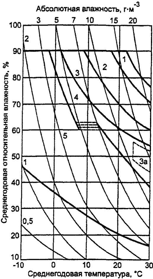
Значения сочетаний "среднегодовая относительная влажность - среднегодовая температура" воздуха для классификационных групп различных типов климатов
